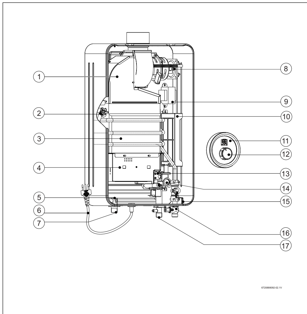
Fig. 3 Construcción del aparato
