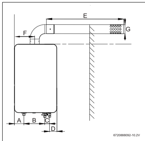
Fig. 10 Dimensiones...(en mm)
