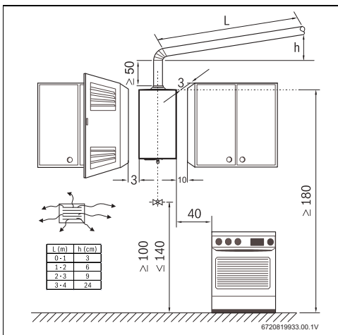
Fig. 13 Separaciones mínimas (en cm)
