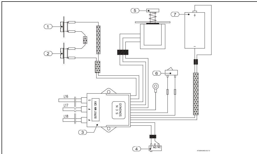
Fig. 4 Esquema eléctrico
