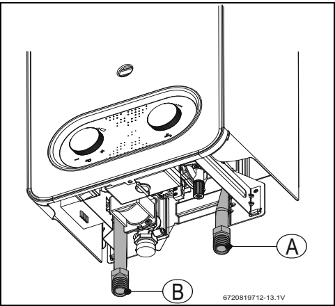
Fig. 14 Tomas de agua
